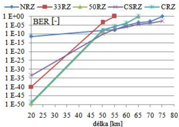
Obr. 8: Závislost chybovosti na délce trasy.
