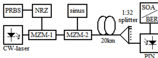
Obr. 3: Blokové schéma konfigurace systému.
