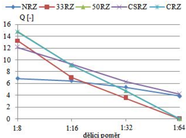
Obr. 7: Závislost Q-faktoru na dělicím poměru splitteru.
