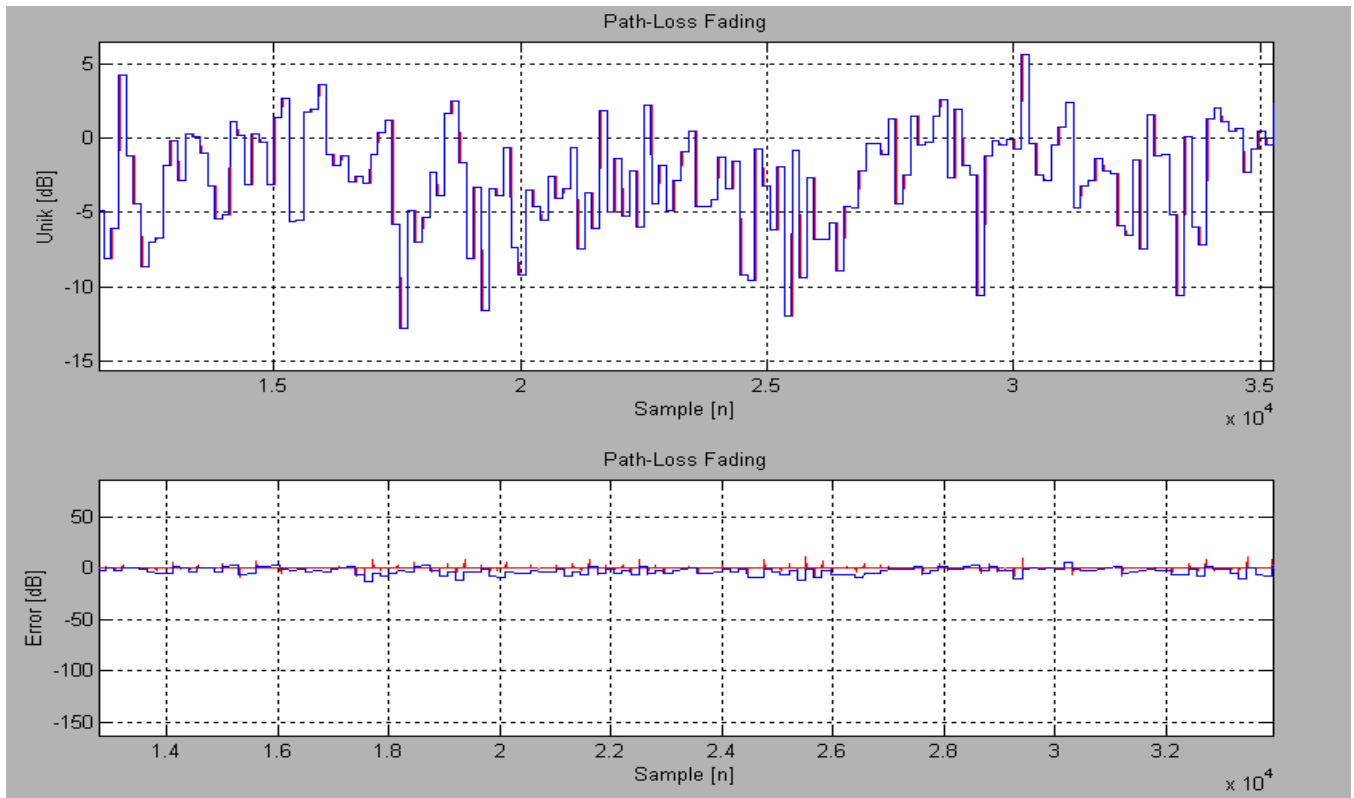
Obr. 3 (hore) Priebeh obálky Rayleighovho simulátora úniku (modrá farba) a jej predikcia pomocou Kalmanovho filtra (červená farba) pre predikčný rozsah 0,41 ms (10 vzoriek).
